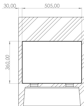
SECCIÓN C-C ESCALA 1 : 7.5
