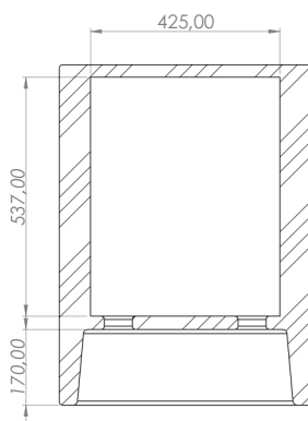
SECCIÓN B-B ESCALA 1 : 7.5
