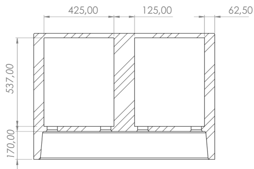
SECCIÓN B-B
