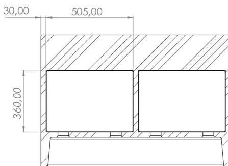
SECCIÓN C-C
